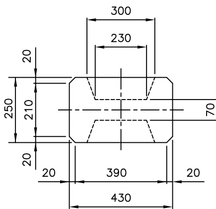
VISTA B-B
